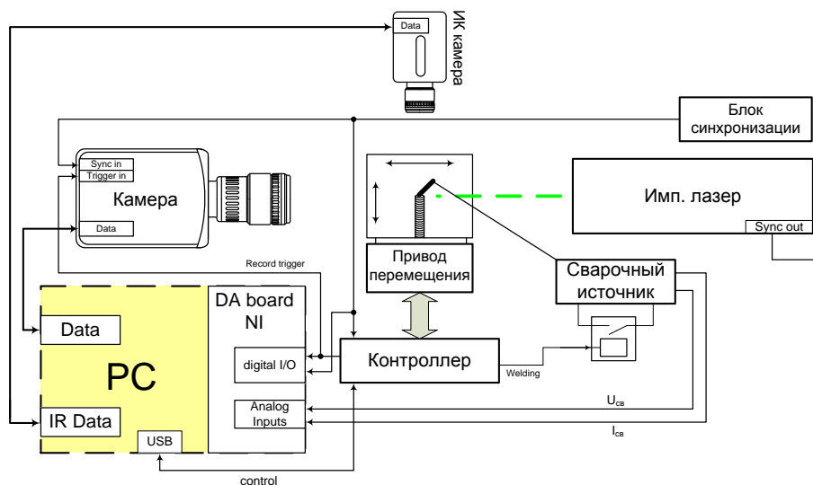
Рисунок 1 – Комплекс для регистрации и исследования быстропротекающих процессов теплопереноса при дуговой сварке плавящимся электродом.
