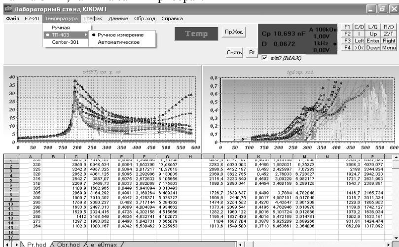
Рисунок 4 – Программа измерений. «Расчет диэлектрической проницаемости и тангенса угла диэлектрических потерь в заданном интервале температур и частот (Лабораторный стенд ЮКОМПИ 3.0)» [2]
