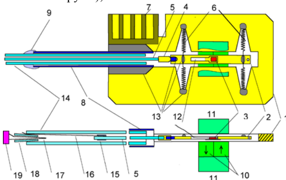
Рисунок 1 – Конструкция дилатометра и датчика перемещения
