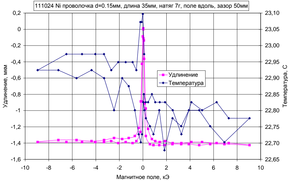
Рисунок 4 – Магнитострикция никелевой проволоки в продольном магнитном поле.
