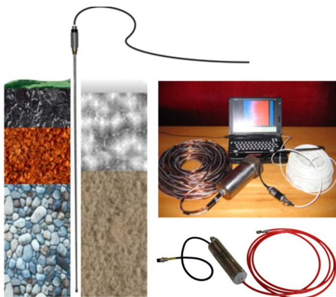
Рисунок 2 – Экспериментальные образцы термопрофилемеров 3,2 м и 50 м для почвы, грунта, льда и осадочных отложений.
