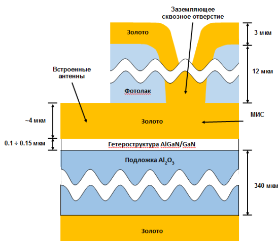
Рисунок 2 – Поперечное сечение пластины с фотолаком
