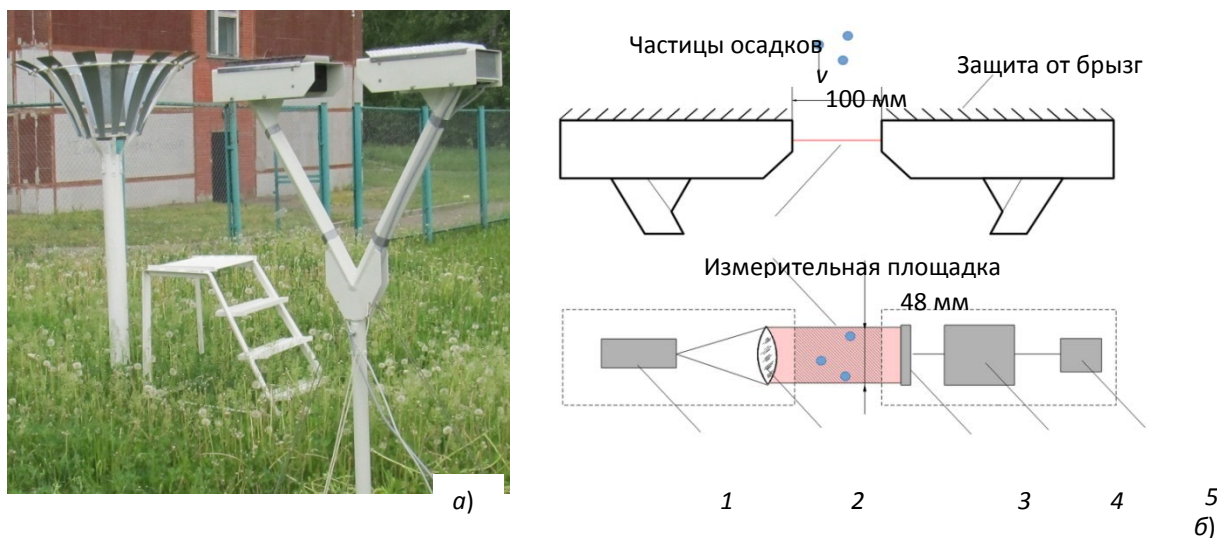
Рисунок 1 – Оптический осадкомер ОПТИОС: а – внешний вид прибора рядом со стандартным осадкомером О-1 на метеорологической площадке ИМКЭС СО РАН; б – функциональная схема ОПТИОС: 1 – источник оптического излучения; 2 – система оптических линз; 3 – линейный сенсор; 4 – блок формирования измерительной информации; 5 – выходной интерфейс.
