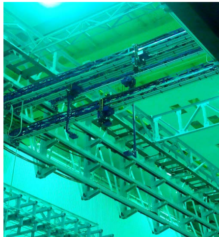
Рисунок 6 – Внешний вид системы обезвешивания солнечной батареей.
