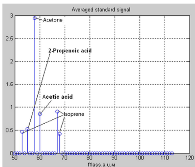
Рисунок 1 – Эталонный масс-спектр
