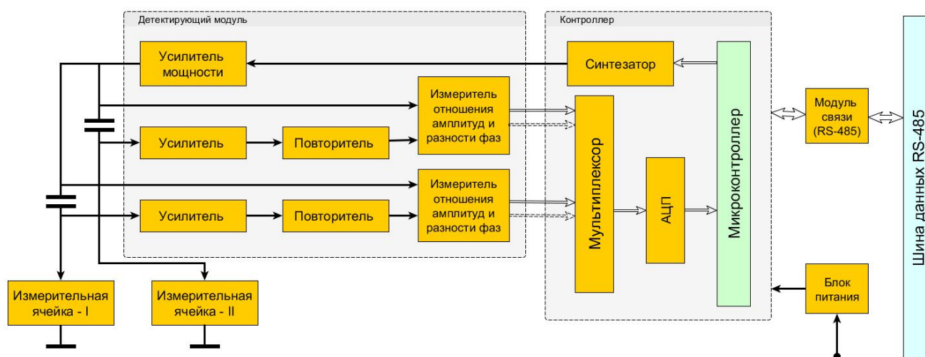
Рисунок 1. Блок-схема скважинного прибора для измерения диэлектрических характеристик пластового флюида
