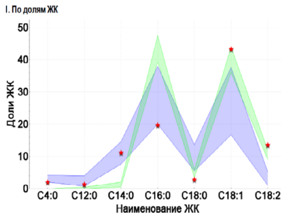
Рисунок 1 – Портативный БИК спектрометр - слева и Протокол определения 7-ми ЖК в среде с его помощью – справа: звездами обозначены доли ЖК, зеленым – поле возможных значений ЖК в пальмовом масле, сиреневым – в молочном жире.
