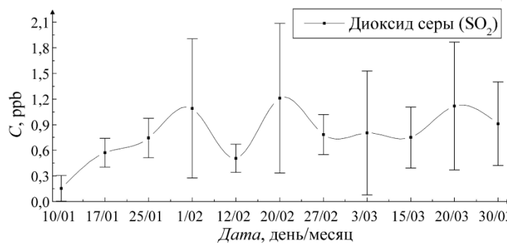
Рисунок 3 – Временной ход содержания диоксида серы
