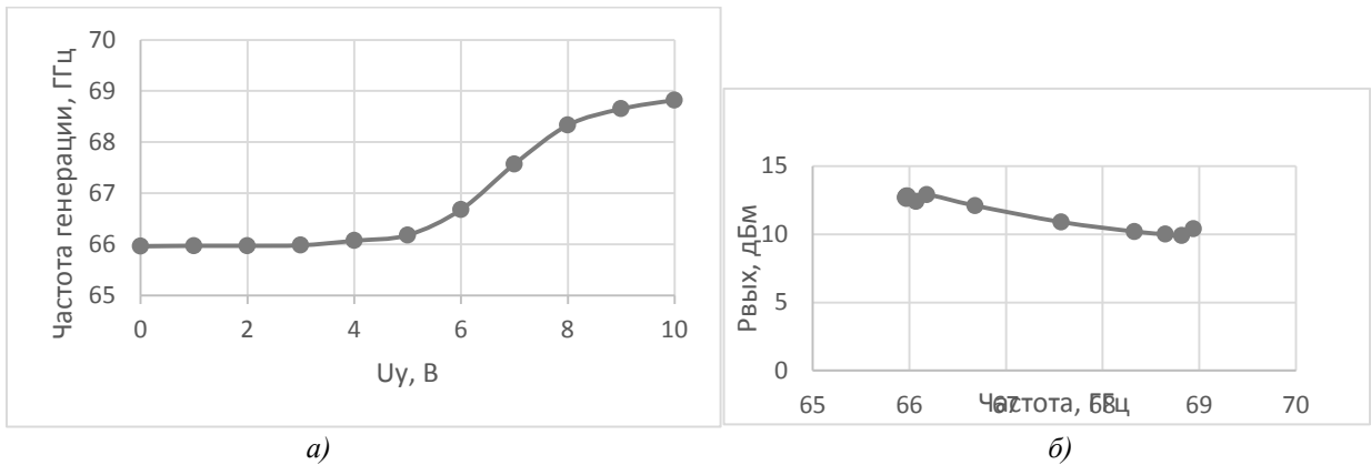
Рисунок 3 – Параметры МИС ГУН - а) зависимость частоты генерации от управляющего напряжения, б) зависимость выходной мощности от частоты
