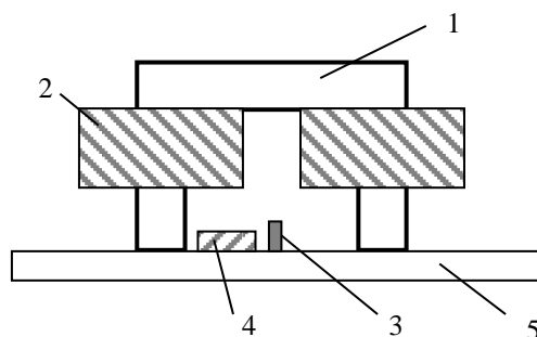
Рисунок 2 – Первичный преобразователь магнитометрического комплекса. 1- магнитопровод, 2 – намагничивающие катушки, 3 – датчик Холла, 4 – накладной вихретоковый преобразователь, 5 – контролируемый образец.
