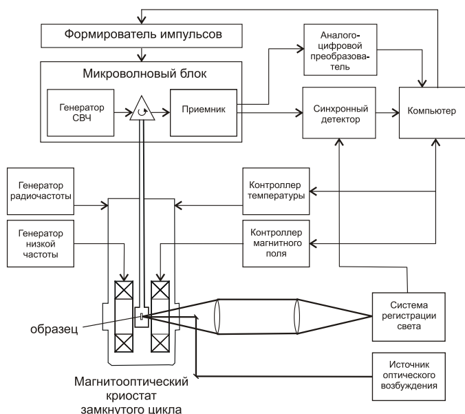
Рисунок 1 – Блок-схема ЭПР/ОДМР спектрометра.
