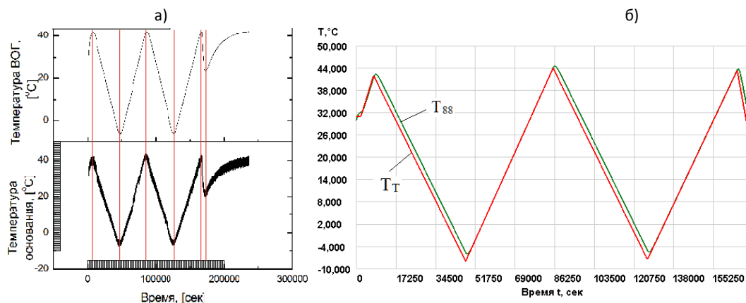
Рисунок 2 – Экспериментальные данные (а) и температура термоплаты ( T_{\gamma} ) и ВОГ ( T_{кк} ) по данным моделирования (б)
