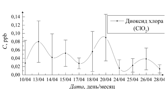
Рисунок 2 – Временной ход содержания диоксида хлора
