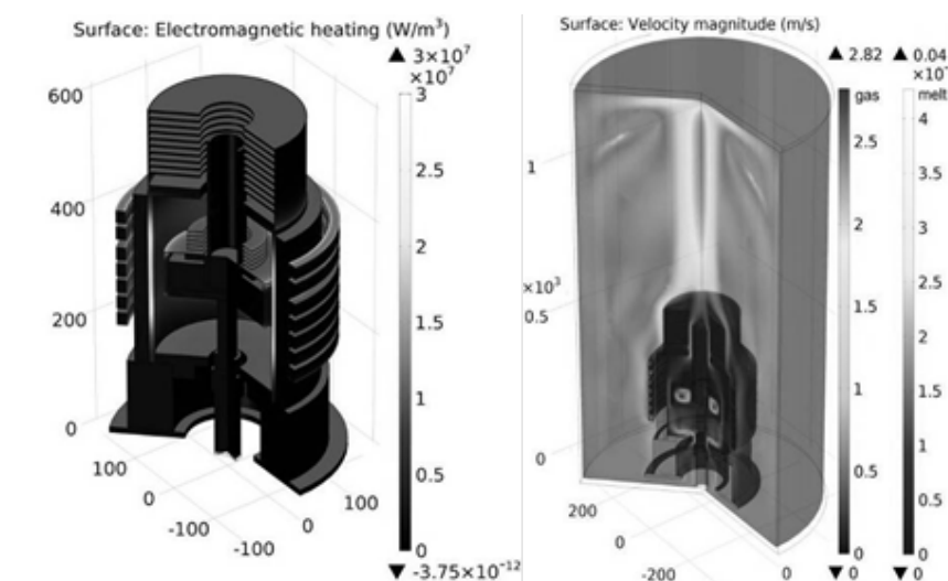
Рисунок 2 – Удельная мощность тепловыделения на элементах теплового узла – (а) и скорости потока газа и расплава – (б)
