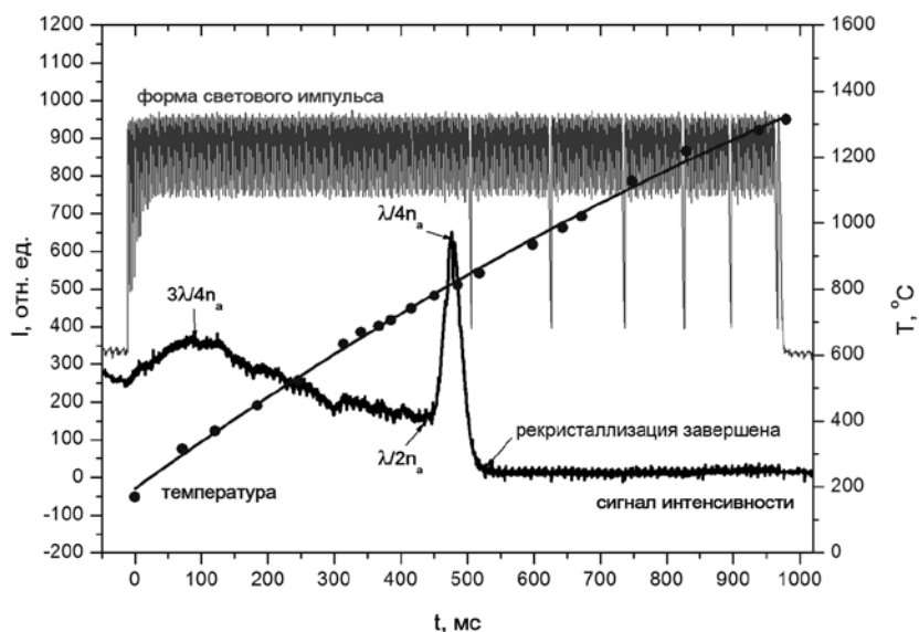
Рисунок 2 – Сигнал изменения интенсивности первого максимума дифракции от амплитудной решетки (а), во время световой импульсной обработки образца импульсом света плотностью мощности 250 \text{ Вт/см}^2 и длительностью 970 мс; форма светового импульса (б).
