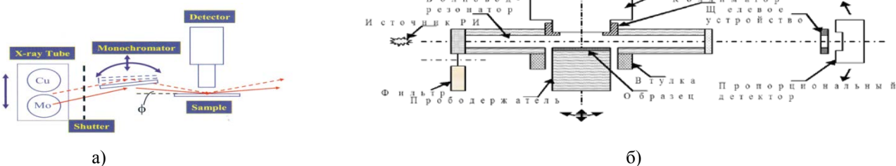
Рисунок 3 – Сравнение традиционной рентгенооптической схемы построения РФА ПВО спектрометра (а) и схемы РФА ПВОВР с расположением образца в волноводно-резонансном канале ПРВР (б).
